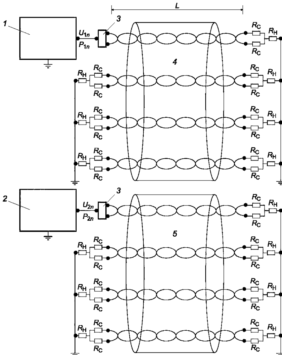
1 — анализатор цепей или генератор сигналов; 2 — анализатор цепей или измерительный приемник; 3 — симметрирующий трансформатор (при необходимости); 4 — влияющий кабель; 5 — подверженный влиянию кабель; R_C и R_H — нагрузка симметричной и несимметричной цепей соответственно; L — длина измеряемых кабелей; P_{1n} ( U_{1n} — мощность (напряжение) сигнала на ближнем конце влияющей пары влияющего кабеля; P_{2n} ( U_{2n} — мощность (напряжение) сигнала на ближнем конце подверженного влиянию пары подверженного влиянию кабеля
