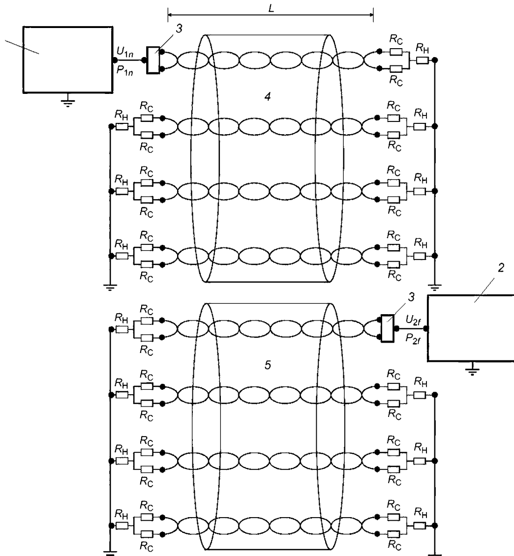
1 — анализатор цепей или генератор сигналов; 2 — анализатор цепей или измерительный приемник; 3 — симметрирующий трансформатор (при необходимости); 4 — влияющий кабель; 5 — подверженный влиянию кабель; R_c и R_H — нагрузка симметричной и несимметричной цепей соответственно; L — длина измеряемых кабелей; P_{yn} ( U_{n\wedge} ) — мощность (напряжение) сигнала на ближнем конце влияющей пары влияющего кабеля; P_{2f} ( U_{2f} ) — мощность (напряжение) сигнала на дальнем конце подверженной влиянию пары подверженного влиянию кабеля
