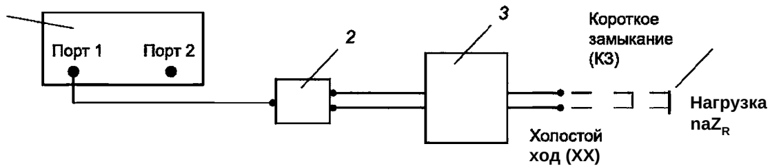
Рисунок 19 — Схема для измерения волнового и входного сопротивлений цепи кабеля и затухания отражения
