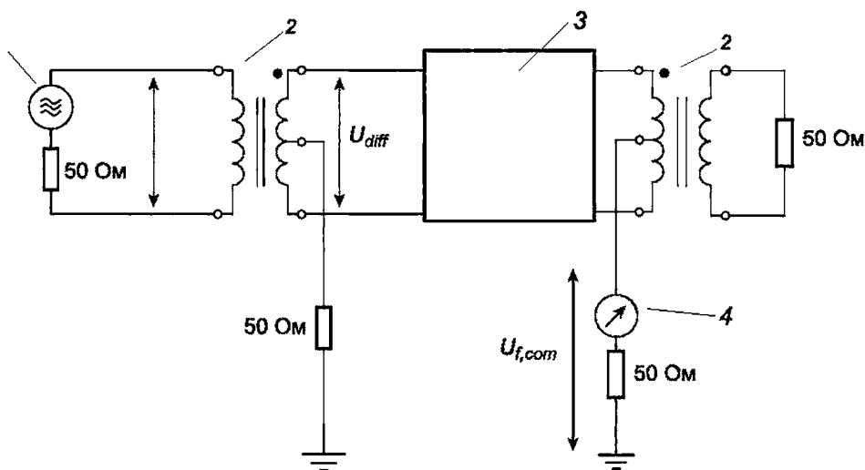
1 — анализатор цепей или временной рефлектометр (ГС); 2 — симметрирующий трансформатор; 3 — измеряемый кабель; 4 — анализатор цепей или временной рефлектометр; U_o — напряжение сигнала на выходе ГС; U_{diff} — напряжение сигнала на ближнем конце симметричной цепи пары кабеля; U_{f,com} — напряжение сигнала на дальнем конце несимметричной цепи пары кабеля
