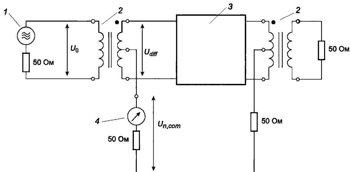
1 — анализатор цепей или временной рефлектометр (ГС); 2 — симметрирующий трансформатор; 3 — измеряемый кабель; 4 — анализатор цепей или временной рефлектометр; U_o — напряжение сигнала на выходе ГС; U_{diff} — напряжение сигнала на ближнем конце симметричной цепи пары кабеля; U_{n,com} — напряжение сигнала на ближнем конце несимметричной цепи пары кабеля
